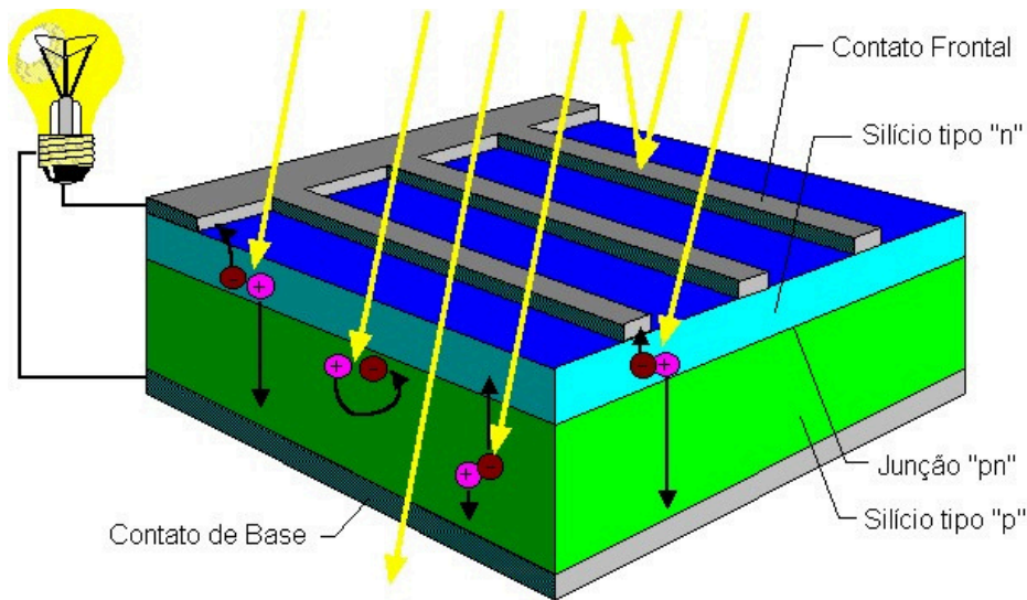
Figura 4.1 - Corte transversal de uma célula fotovoltaica
