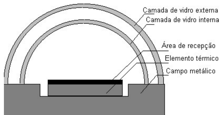
Figura 3.2 - Secção transversal de um piranômetro
