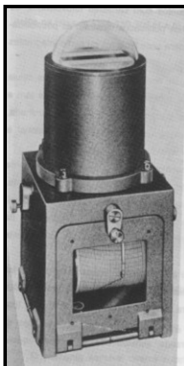
Figura 3.6 - Actinógrafo Robitzsch- Fuess
